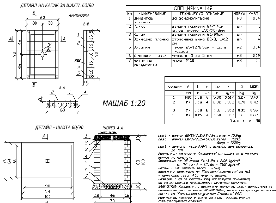
Фигура - Кабелна шахта – единична
